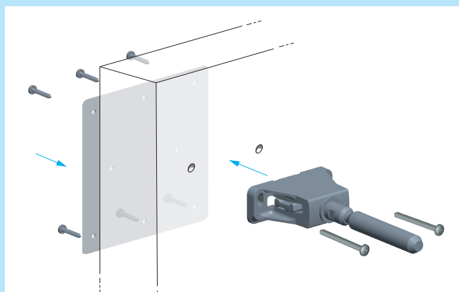
1. FISSARE LA PIASTRA SUL RETRO DEL PANNELLO CON VITI PANELVIT TC Ø3.5.
