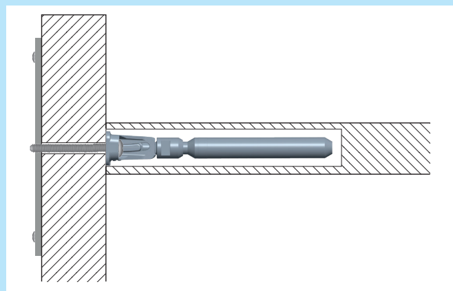
2. FISSARE TRIADE ALLA PIASTRA ATTRAVERSO I FORI PREDISPOSTI NEL PANNELLO TRAMITE VITI TC M5.
