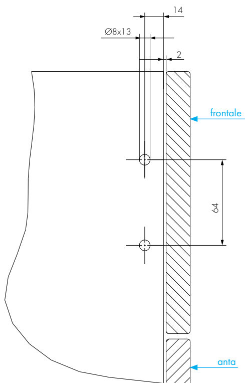
FORATURA FIANCO
