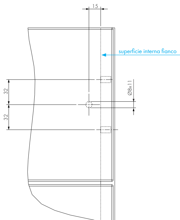
FORATURA FRONTALE
